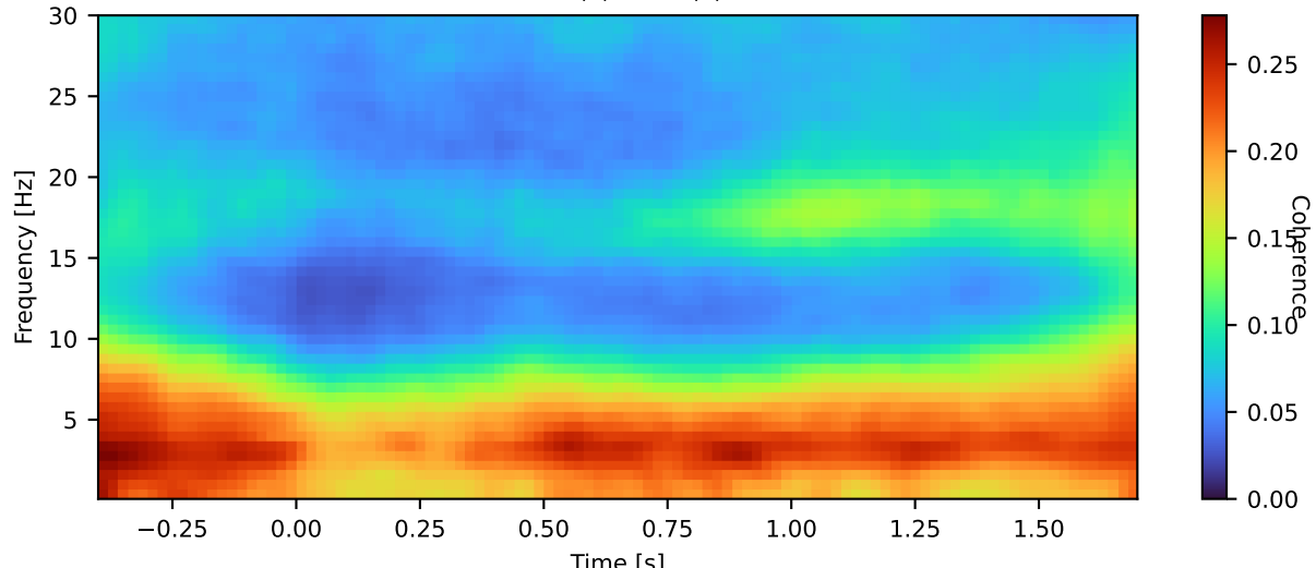
dPFC (0) - 8AD (1)
